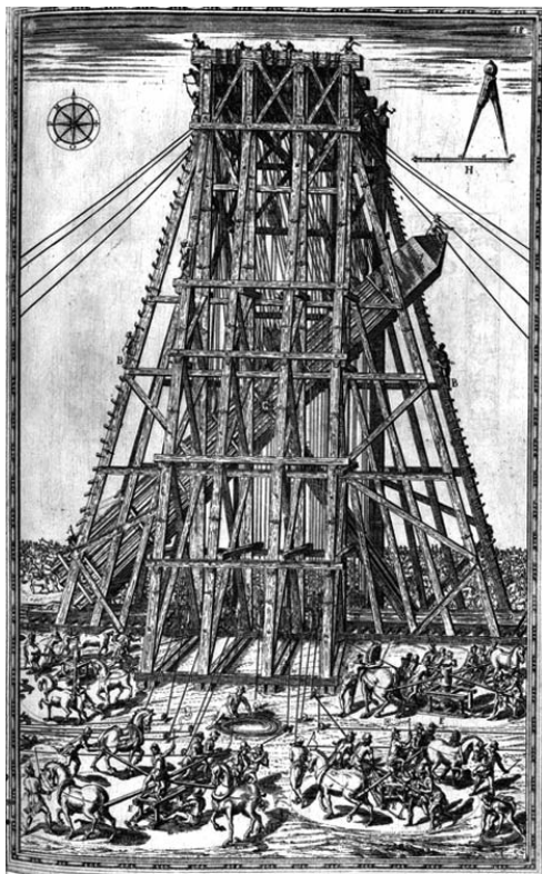
Podizanje vatikanskog obeliska (prema starom crtežu)
