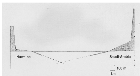
Slika 65: Izmereni nagibi (pune linije) duž Akabskog zaliva kod Nuveibe. Zapazite da je nagib grafički preterano izražen na slici. Ako bi se takav nagib prostirao preko celog zaliva maksimalna dubina bi iznosila oko 240 m (tačkaste linije).
