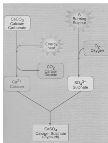
Slika 13: Verovatna šema hemijskih reakcija nesreće koja je pogodila ovo mesto. \text{CaCO}_3 , Kalcijum karbonat; S, Gorući sumpor; Energija (toplota), \text{O}_2 , Kiseonik; \text{CO}_2 , Ugljen-dioksid; \text{Ca}^{2+} , Kalcijum; \text{SO}_4^{2-} , Sulfat; \text{CaSO}_4 , Kalcijum sulfat (Gips).
