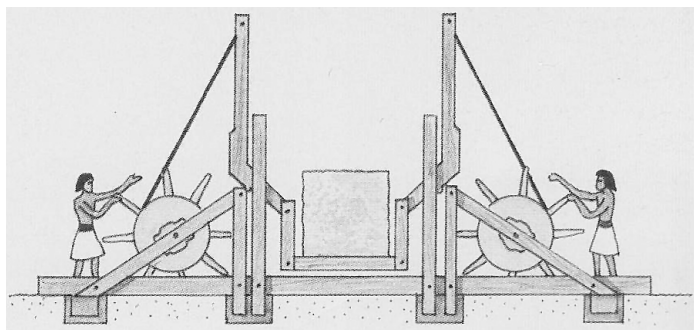
Slika 36: Osnovni princip naprave za podizanje izgrađene za podizanje teških komada stena. Rupe u zemlji su služile za stabilizaciju cele konstrukcije (videti slike 207-211).
